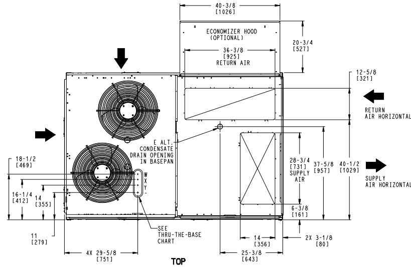
TOP
